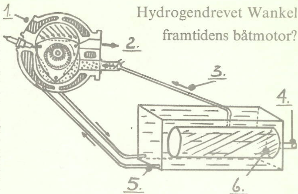
Blir dette framtidens motorinstallasjon? Amerikanske forskere mener så. Skissen viser prinsippet for Wankel-motor med hydrogendrift. 1) Wankel-motor. 2) Avgass. 3) Hydrogen til motor. 4) Påfylling av hydrogen. 5) Kjølevann fra motor for oppvarming. 6) Metallhydrid for absorbering av hydrogen.
